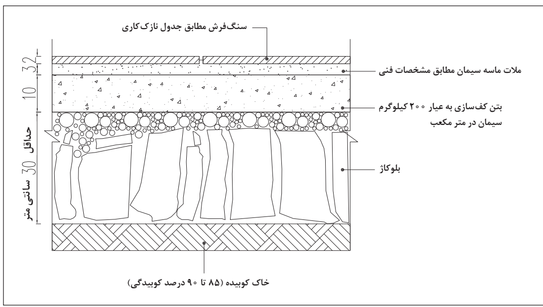
جزئیات اجرای سنگ روی خاک
